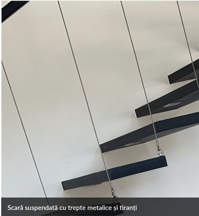
Detaliu prindere tiranți și treaptă metalică
